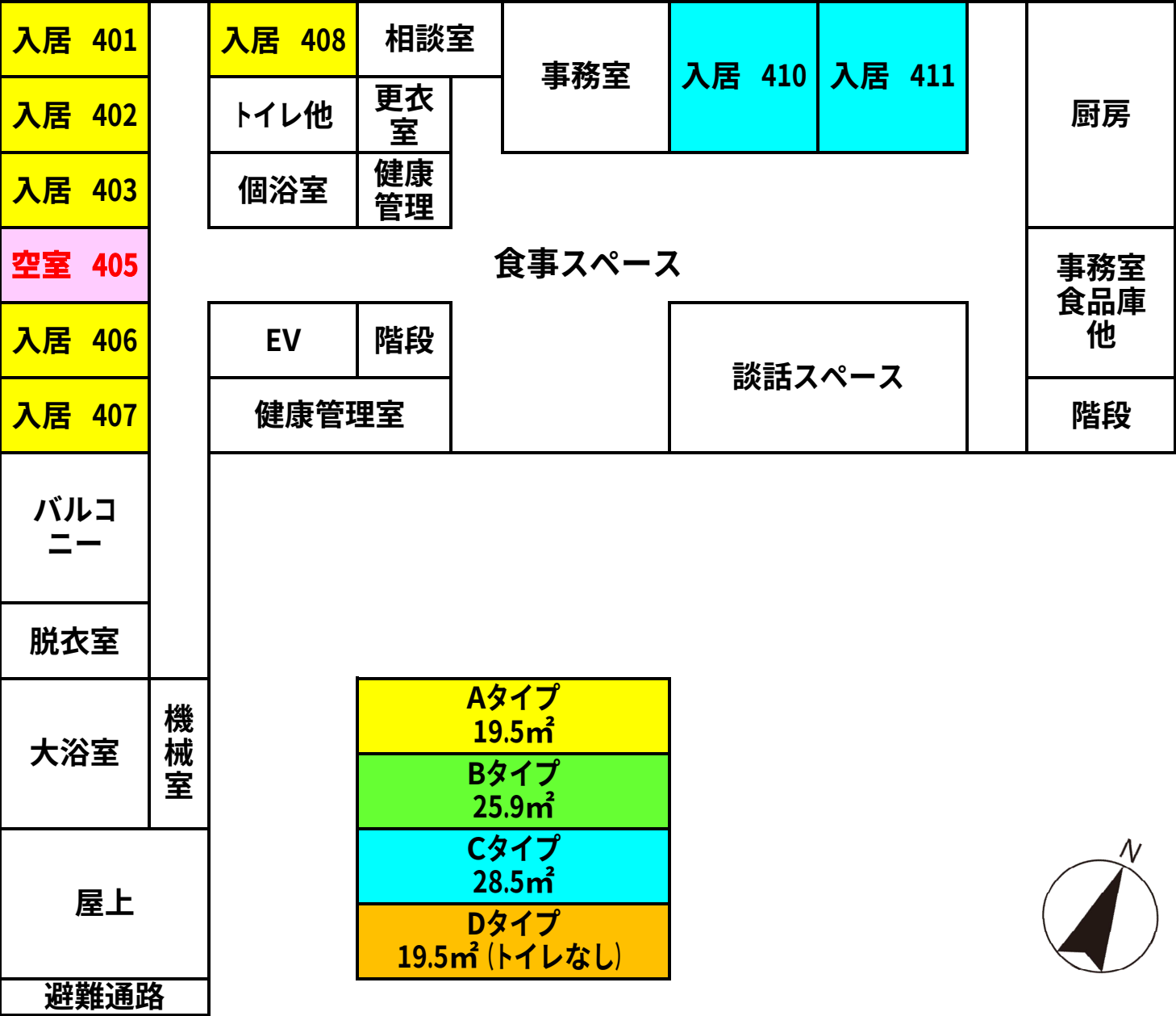
有料老人ホームチエロ平面図 4階
